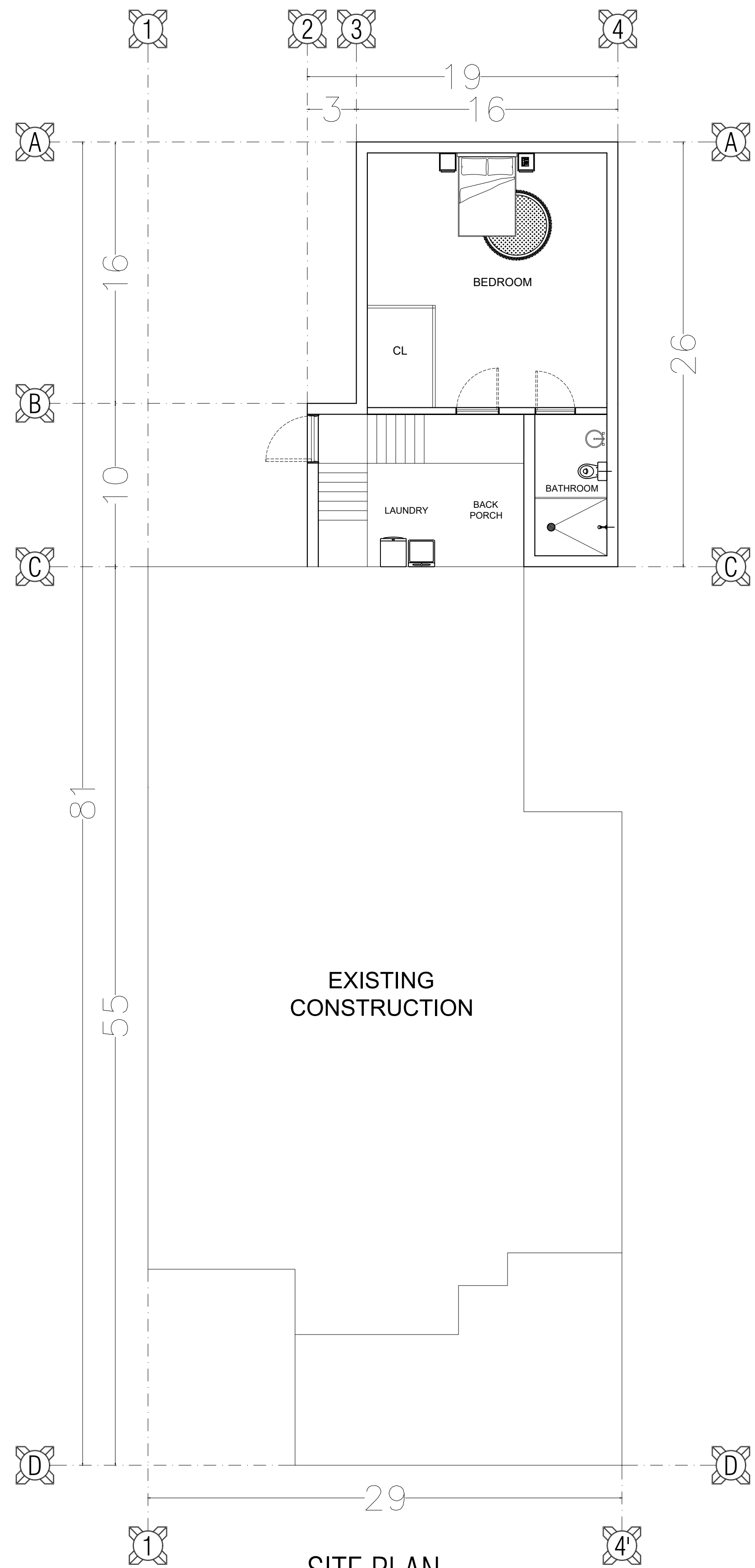
SITE PLAN ESC 1:100 [ft]
